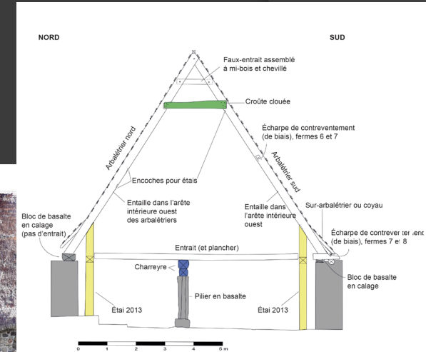
Relevé en coupe d'une ferme de la charpente
